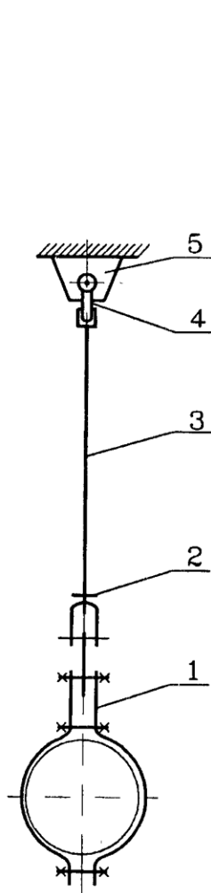
1 – узел крепления; 2 – гайка; 3 – тяга резьбовая; 4 – вилка; 5 – проушина
