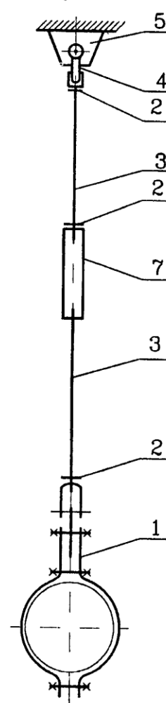
1 – узел крепления; 2 – гайка; 3 – тяга резьбовая; 4 – вилка; 5 – проушина; 7 – талреп
